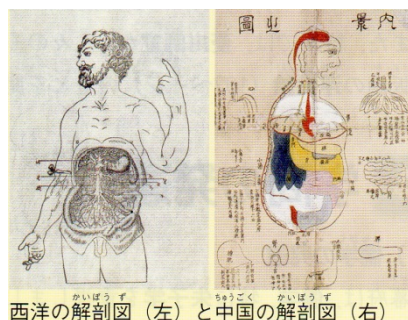
西洋の解剖図 (左) と中国の解剖図 (右)
