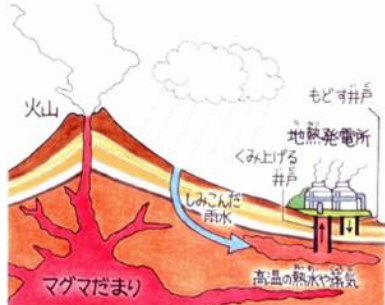
地熱発電のしくみ
